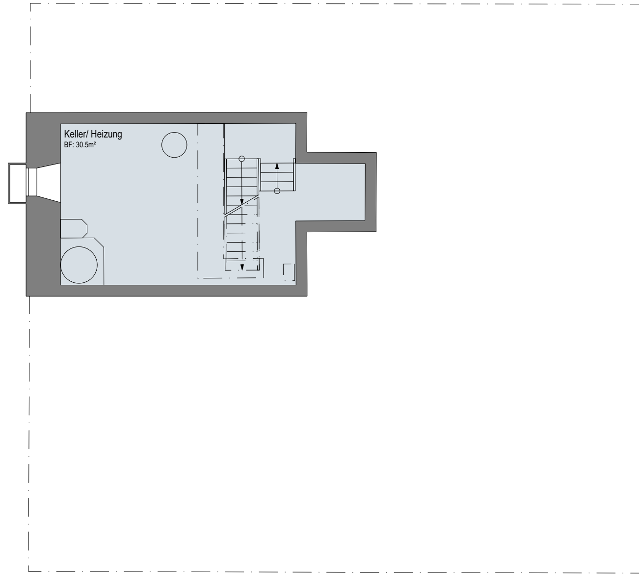
Untergeschoss 1:100
