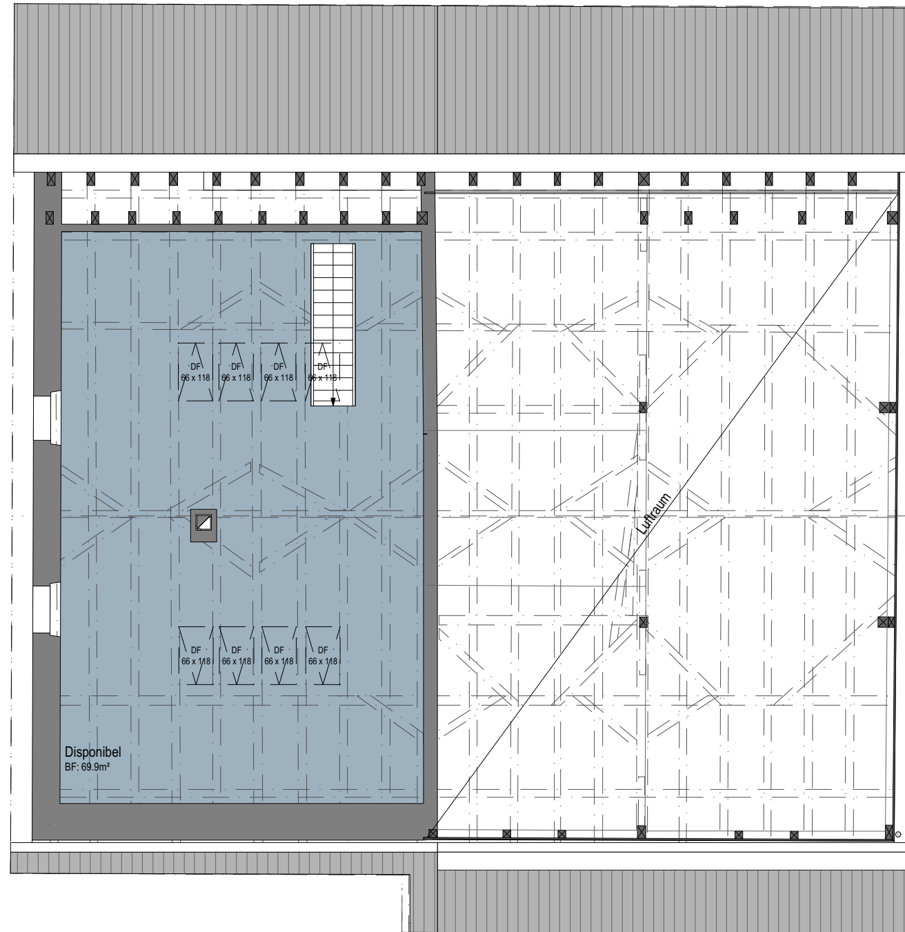
Dachgeschoss 1:100
